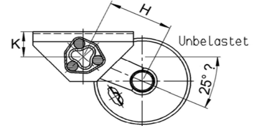
Schnitt A-B Bowdenzug unten angeschlagen
